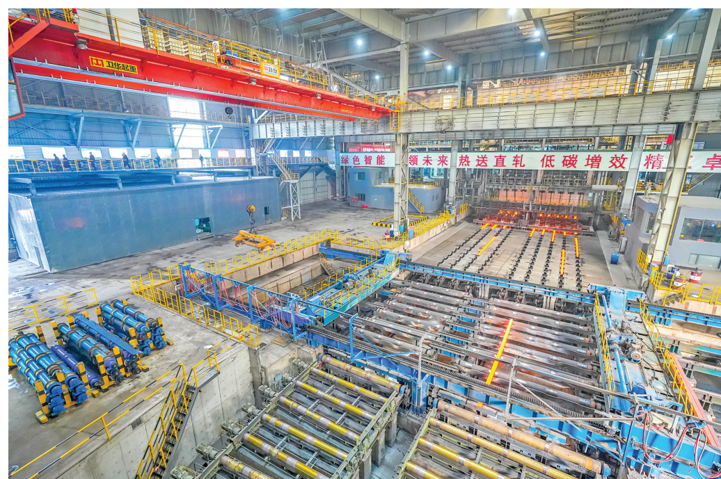
2月8日,河津宏达钢铁集团有限公司自动化生产线满负荷运转,加速生产订单产品,力争实现一季度“开门红”。近年来,河津市持续做大做强精品钢铁产业基地,通过提升装备水平、完善产能配套、延伸产业链条,打造智慧型绿色低碳增效工厂,为工业经济发展壮大注入了活力,增添了动力。本报记者 闻鑫奇 摄影报道
