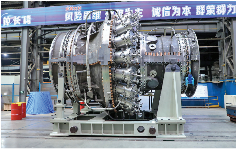
2023年6月4日，中国航发“太行110”重型燃气轮机(代号AGT-110)在深州通过产品验证鉴定。 新华社发
