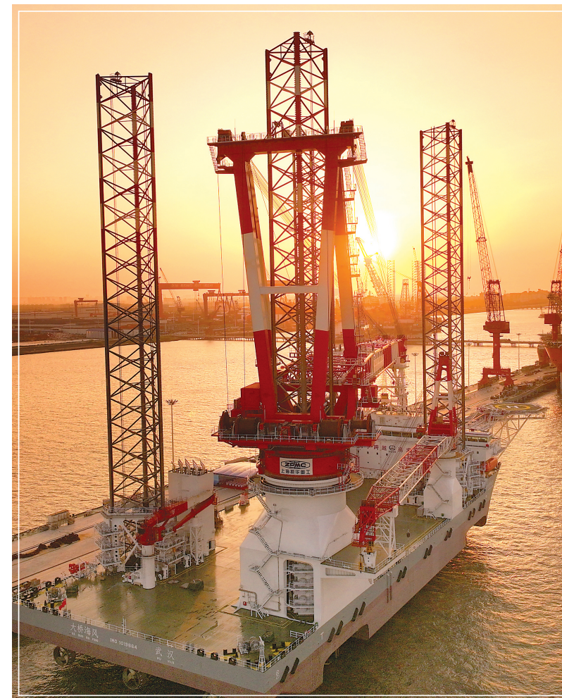
5月18日拍摄的晨光中的“大桥海风”号(无人机照片)。当日，由中铁大桥局和招商工业共同研制的最新一代2000吨自升式海上风电安装平台“大桥海风”号在江苏南通交付。“大桥海风”船长138米，船宽53米，拥有4根131米高的桩腿，多项性能指标达到国际领先水平。 新华社发(许丛军 摄)
