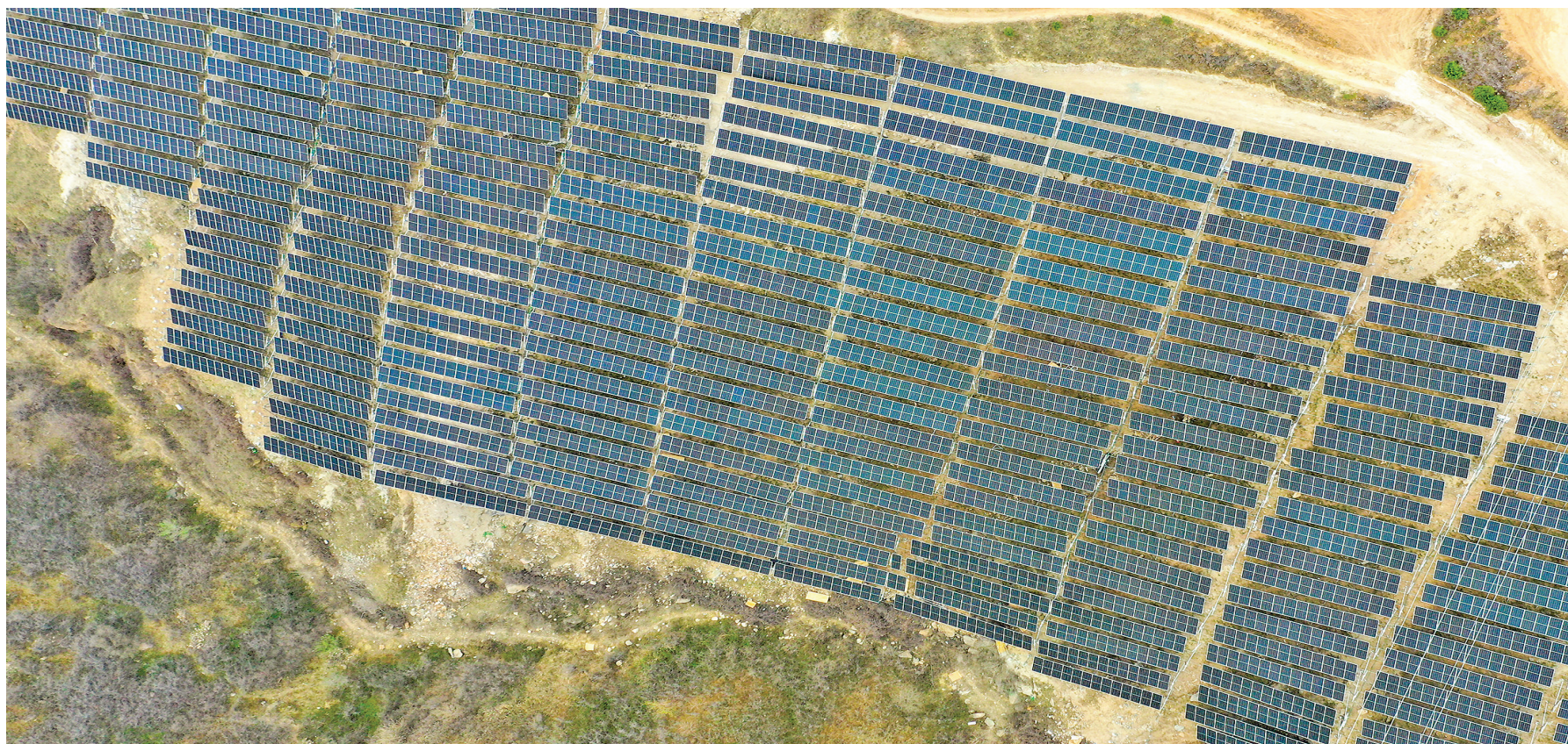
3月26日,夏县瑶峰镇境内的陕煤电力光伏发电项目现场,光伏板整齐地排列在山坡上。据了解,总投资4.67亿元的100MW光伏发电项目,是当地政府引进的清洁能源企业。项目建成后,预计年发电量1.54亿千瓦时,年产值约5100万元,有力推动县域经济社会可持续发展。 特约摄影 张秀峰 摄
