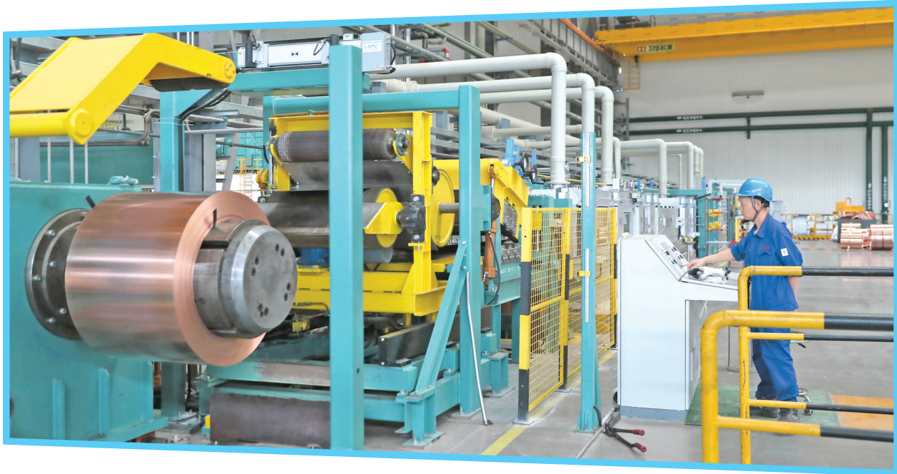
▲山西北铜新材料科技有限公司生产车间
