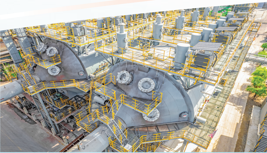
▲山西建龙集团热轧流程智能“循环碳”项目
